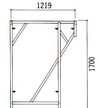
ブラケット枠 B-9012
