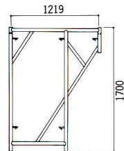
ブラケット枠 B-7612
