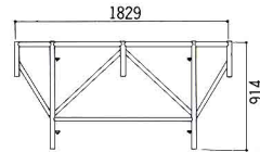
支保工枠 KB-9109
