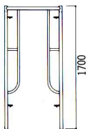
鳥居型枠 A-2655A
