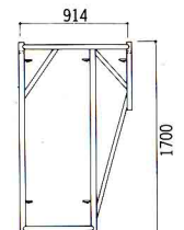
ブラケット枠 B-6190
