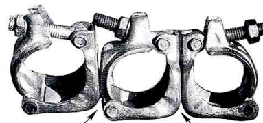
三ヶ連自在クランプ 3C-48F
