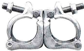
自在クランプ C-48F
