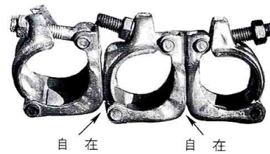
三ヶ連自在クランプ 3C-48F (48.6φ×48.6φ×48.6φ) ●許容荷重…3.43kN ●質量…1.0kg (350kg)
