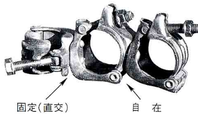
三ヶ連直交クランプ 3C-48C (48.6φ×48.6φ×48.6φ) ●許容荷重…4.90kN ●質量…1.1kg (500kg)
