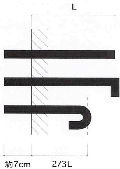
アンカーボルトの長さについて
