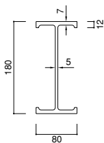
(断面性能)
